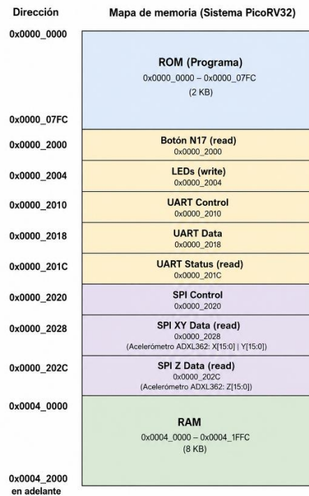
Figura 3. Mapa de memoria
