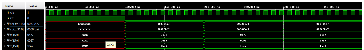
Figura 4. Testbench del módulo spi_adxl362.
