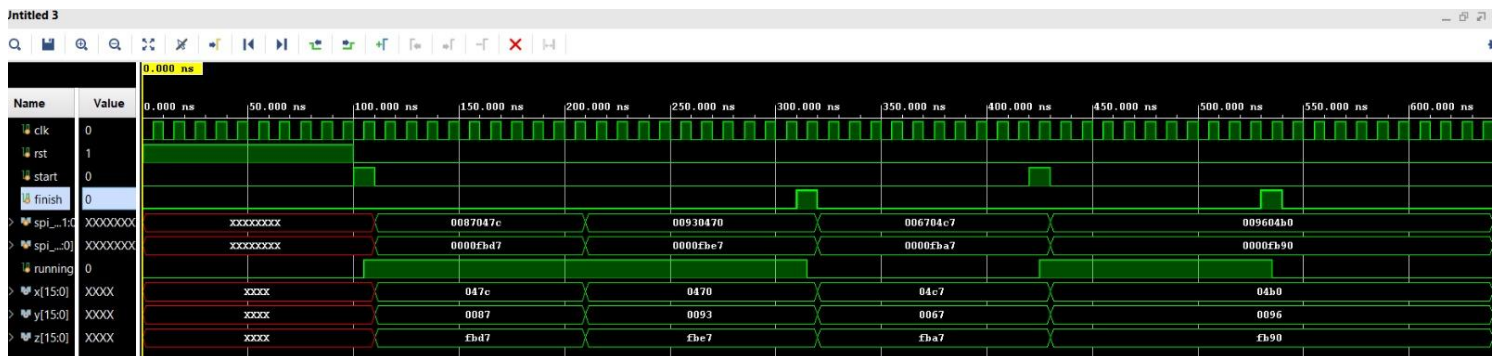
Figura 4. Testbench del módulo spi_adxl362.
